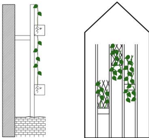
72–73. ábra Homlokzattól független állványrendszerrel, támszerkezetre futtatott kúszónövényvel kialakított zöldhomlokzat (jellegábrák) (Pataky–Csibi)
