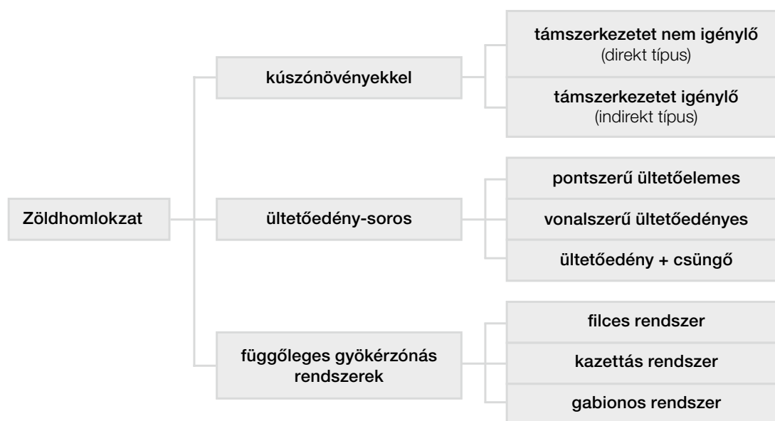
42. ábra Zöldhomlokzatok rendszerezése (Pataky)
